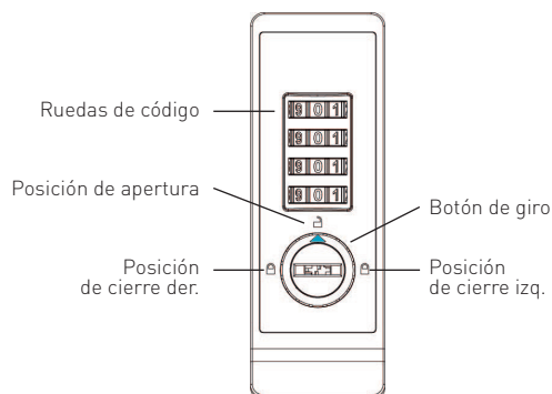
Vista delantera de la cerradura
