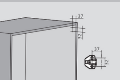
Sistema de bisagras de Doble Orificios
