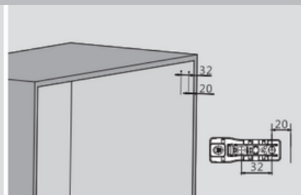
Sistema de bisagras base recta
