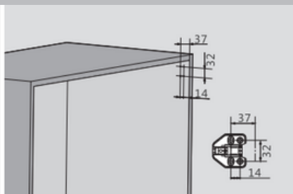
Sistema de bisagras de Cuatro Orificios
